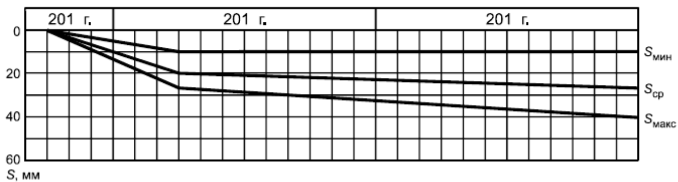
Рисунок Г.4 - График развития перемещений
