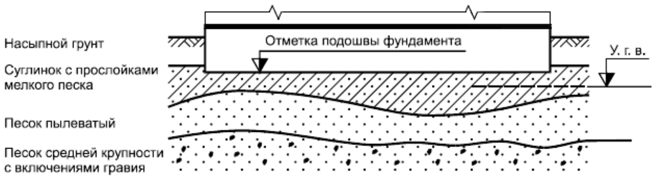
Рисунок Г.1 - Схема фундамента и основания
